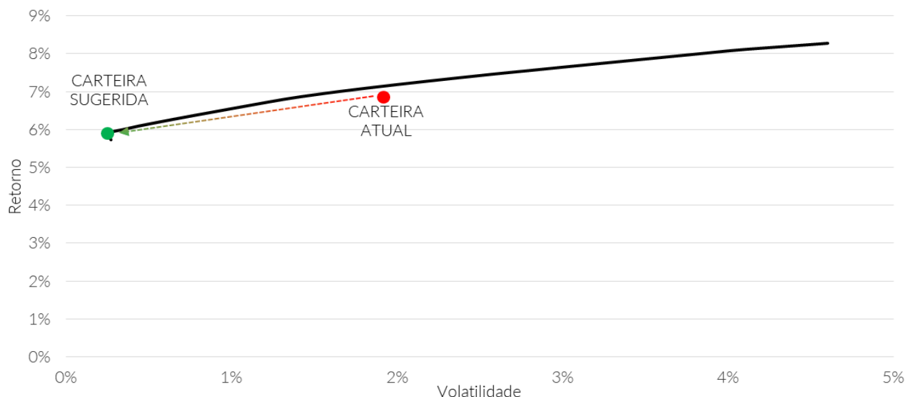
Figura 6 - Fronteira eficiente de Markowitz
